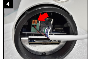
4 Orangene Klemmen eindrücken, um die Federung zu lösen und Spannungs-Adern herausziehen.
