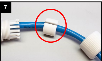
7 Kabel durch den seitlichen Schlitz in die Dichtung pressen.
