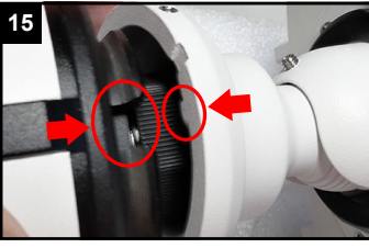
15 Kerbe an der Kamera muss in die Wölbung am Wandarm einrasten.
