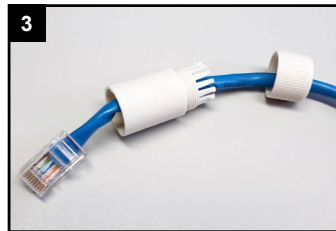
Verschraubung und Schraub-bolzen über das Kabel ziehen.
