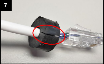
7 Dichtungsring über den seitlichen Schlitz entfernen.
