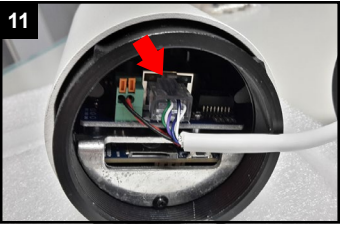
11 Netzwerksstecker in der Kamera anschließen.
