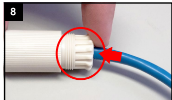
8 Dichtung in den Schraubbolzen pressen.
