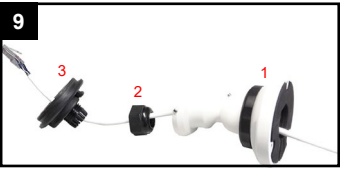
9 Neue Kabel nacheinander durch Halter, Kabelverschraubung und durch Rückwand ziehen.
