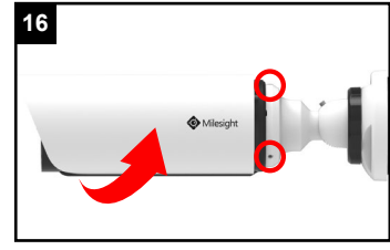
16 Kamera ein wenig drehen zum Einhaken. Drei Madenschrauben an der Halterung feste anziehen.
