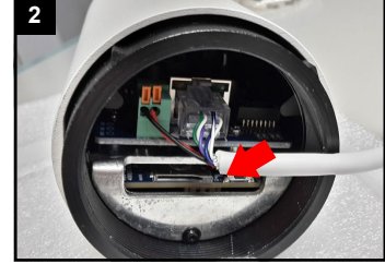
2 Für Reset: Fünf Sekunden lang die Taste gedrückt halten.
