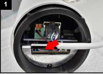
1 Der Kartenslot befindet sich hinter der Rückwand.
