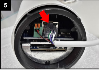
5 Netzwerkstecker an der Klemme eindrücken und herausziehen.
